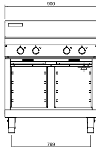
IN514F
